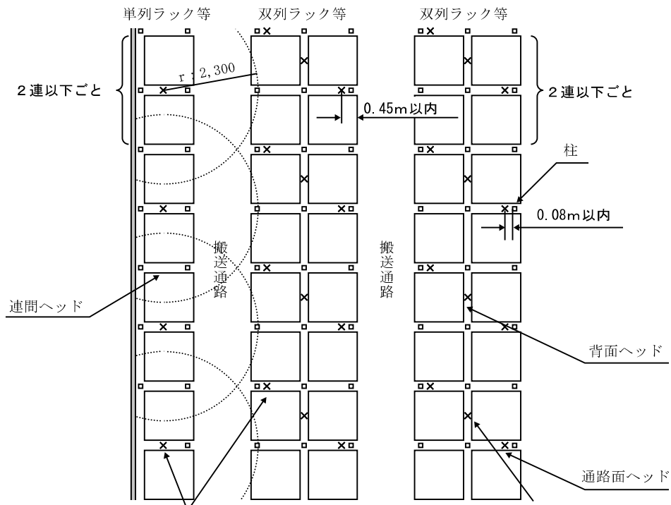
第3の4-8図
