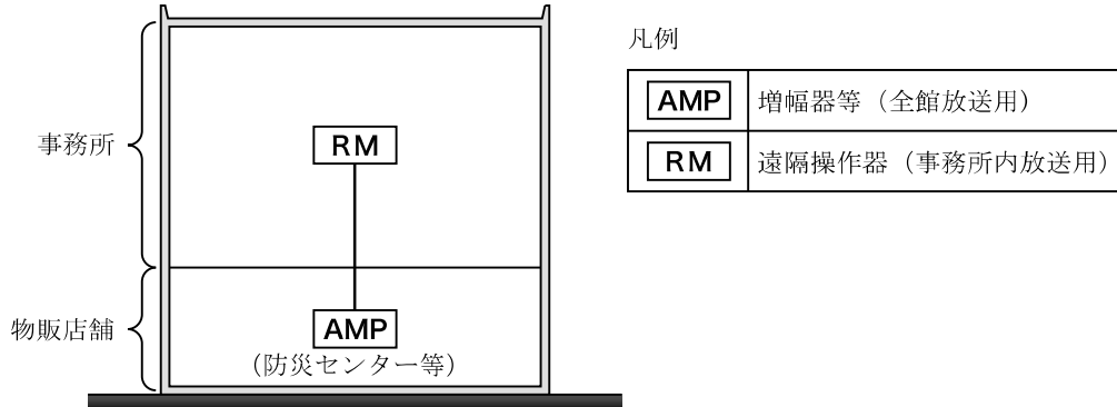
（避難が防火対象物の部分ごとに独立して行われると考えられる場合の例 (イ)関係）
